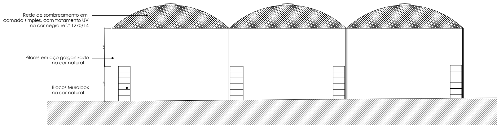
ALÇADO POENTE
