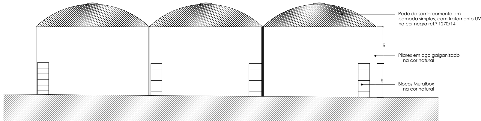
ALÇADO NASCENTE
