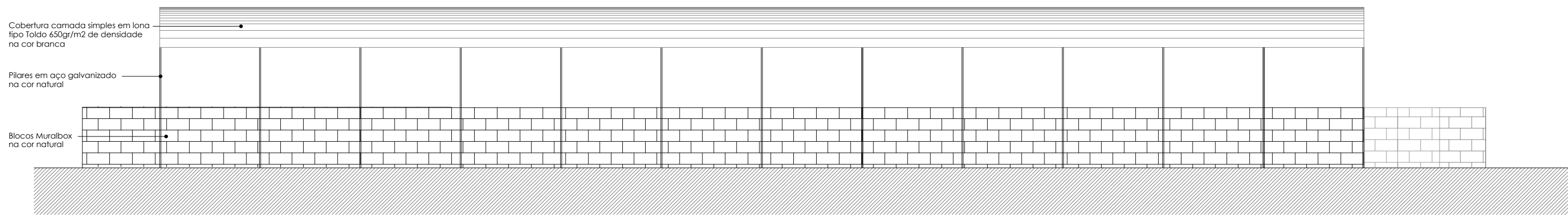
ALÇADO SUL
